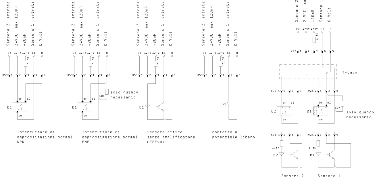
Connessione del sensore
